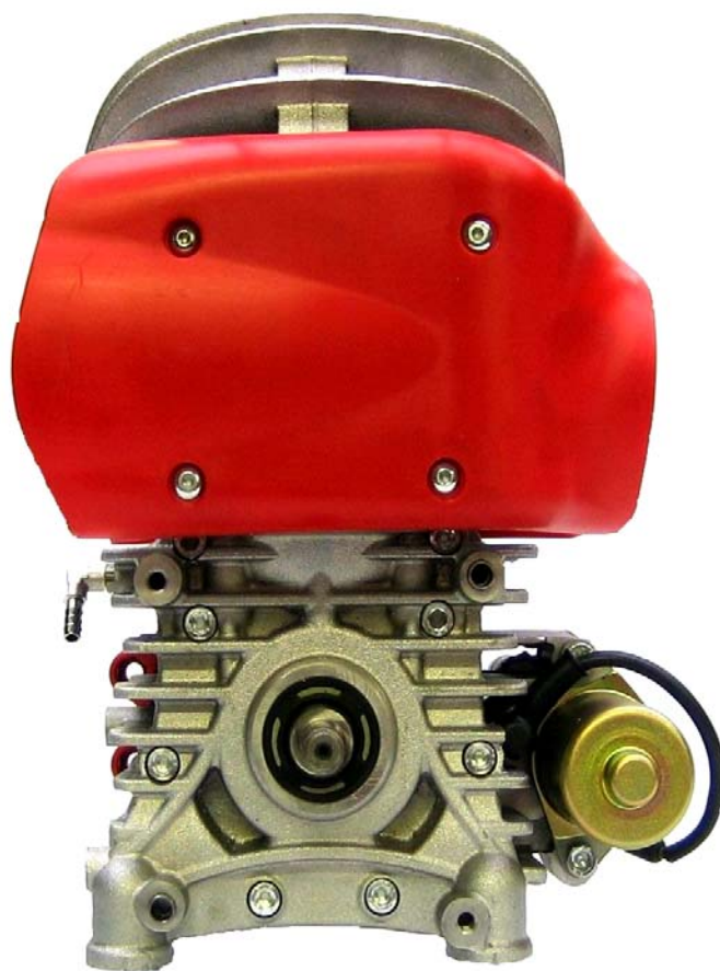
FOTO DEL MOTORE – LATO OPPOSTO
