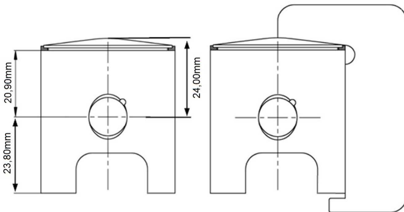
Photo du piston (de l'avant, de côté et d'en haut) / Photo of the piston (front, side and top)
